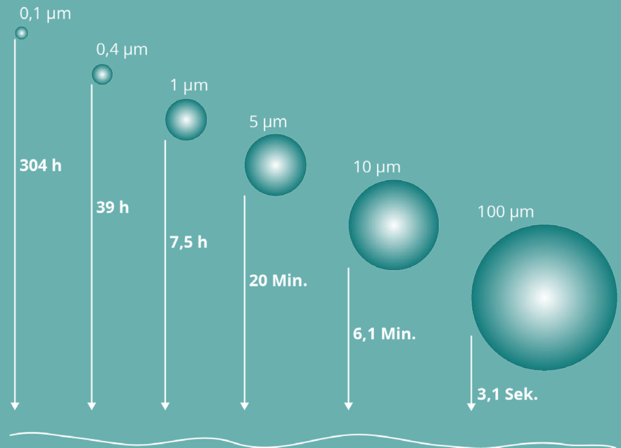
Abbildung 2: Beispielhafte Darstellung der durch die Schwerkraft bedingten Sedimentation kugelförmiger Partikel mit der Dichte 1\text{ g/cm}^3 in ruhender Luft *Abbildung nicht maßstabsgetreu
